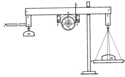
Schéma du dispositif d'essai de G.A.Hirn (1854)
